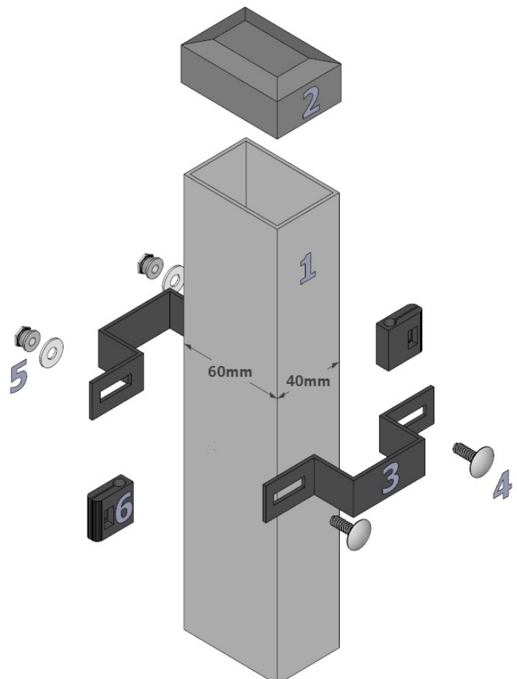
OBEJMA NAROŻNA
